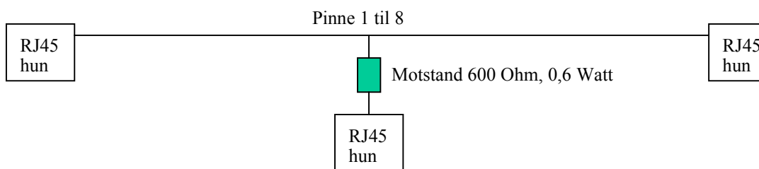
Prinsippskisse/koblingsskjema
